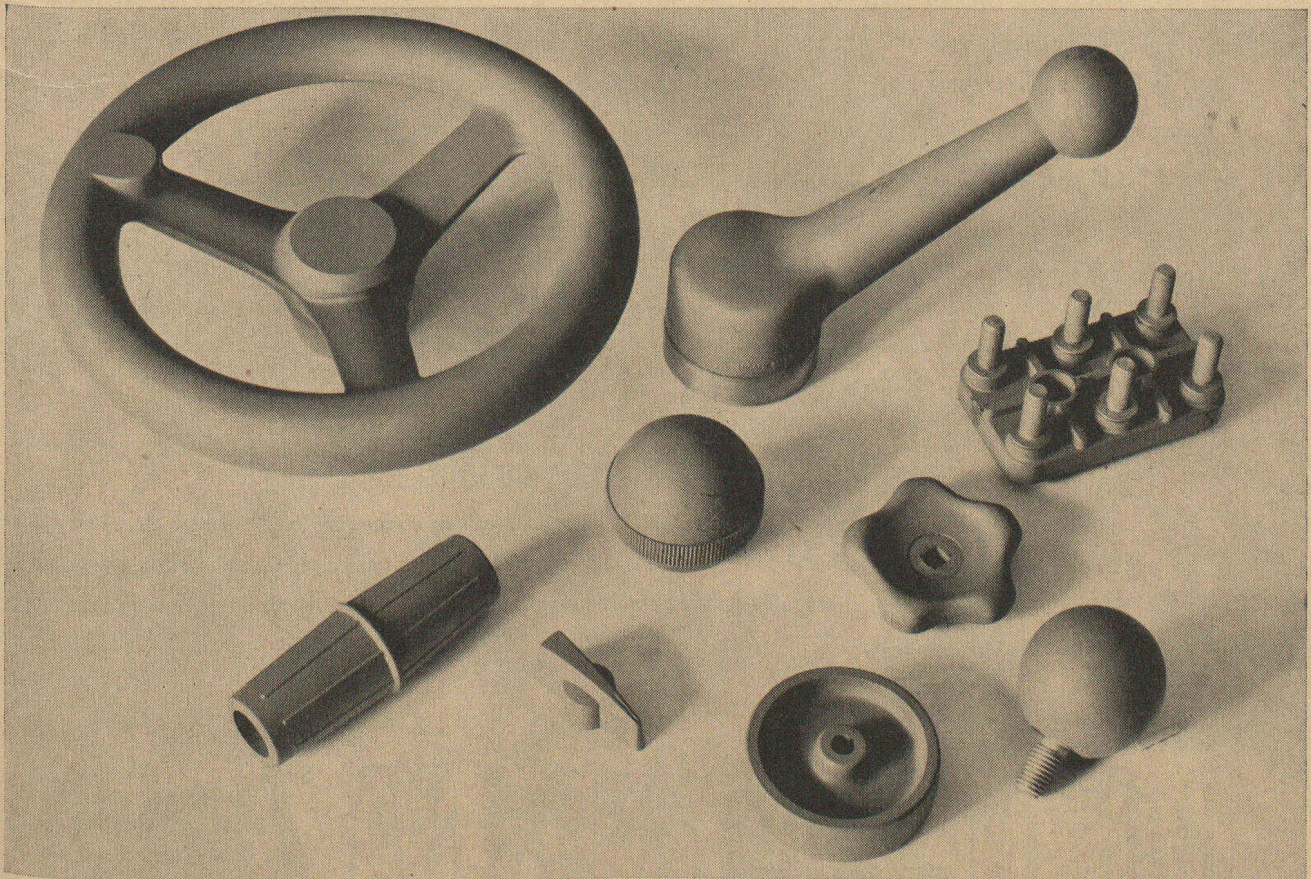
Quelques pièces standard en matière synthétique (Résoforme) fabriquées par Micafil S. A., Zurich, pour l'équipement de machines-outils.
