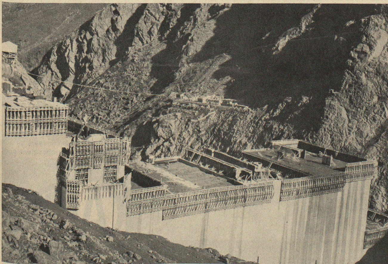
Barrage de la Grande Dixence avec BARRA 55 - Vinsol. — Première étape 1'800'000 m 3
