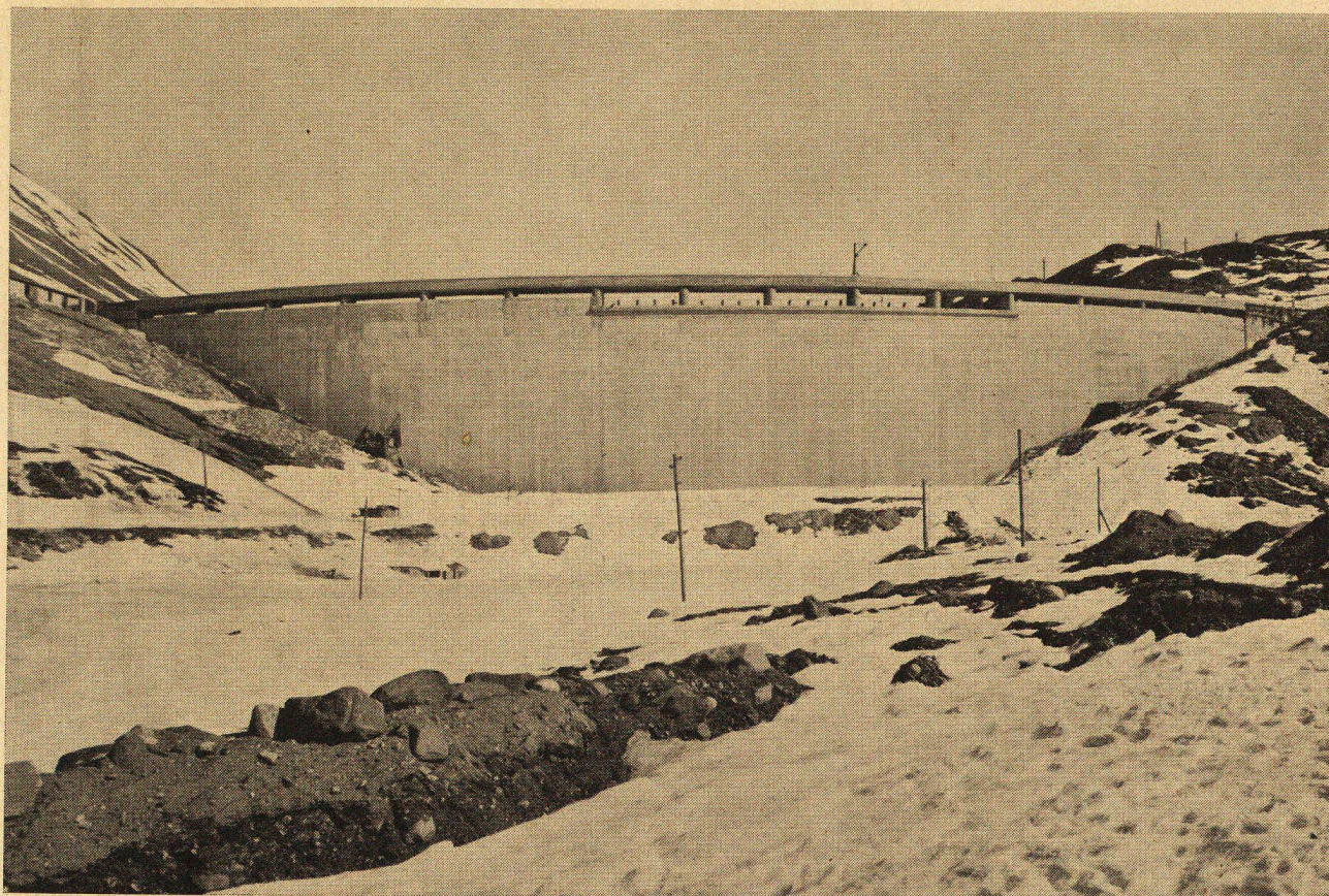
Barrage de Margaritze, de la Tauernkraftwerke, Glockner-Kaprun. — Béton au FRIOPLAST
