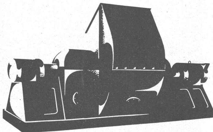
Ventilateur de tirage induit pour une installation de chaudières, Q = 72 \text{ m}^3/\text{s} ; p = 220 \text{ mm eau}
