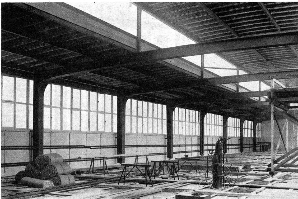
Halles IIb et IIIb de la Foire de Bâle Isolation thermique des toitures par matelas VETROFLEX « Construction »
