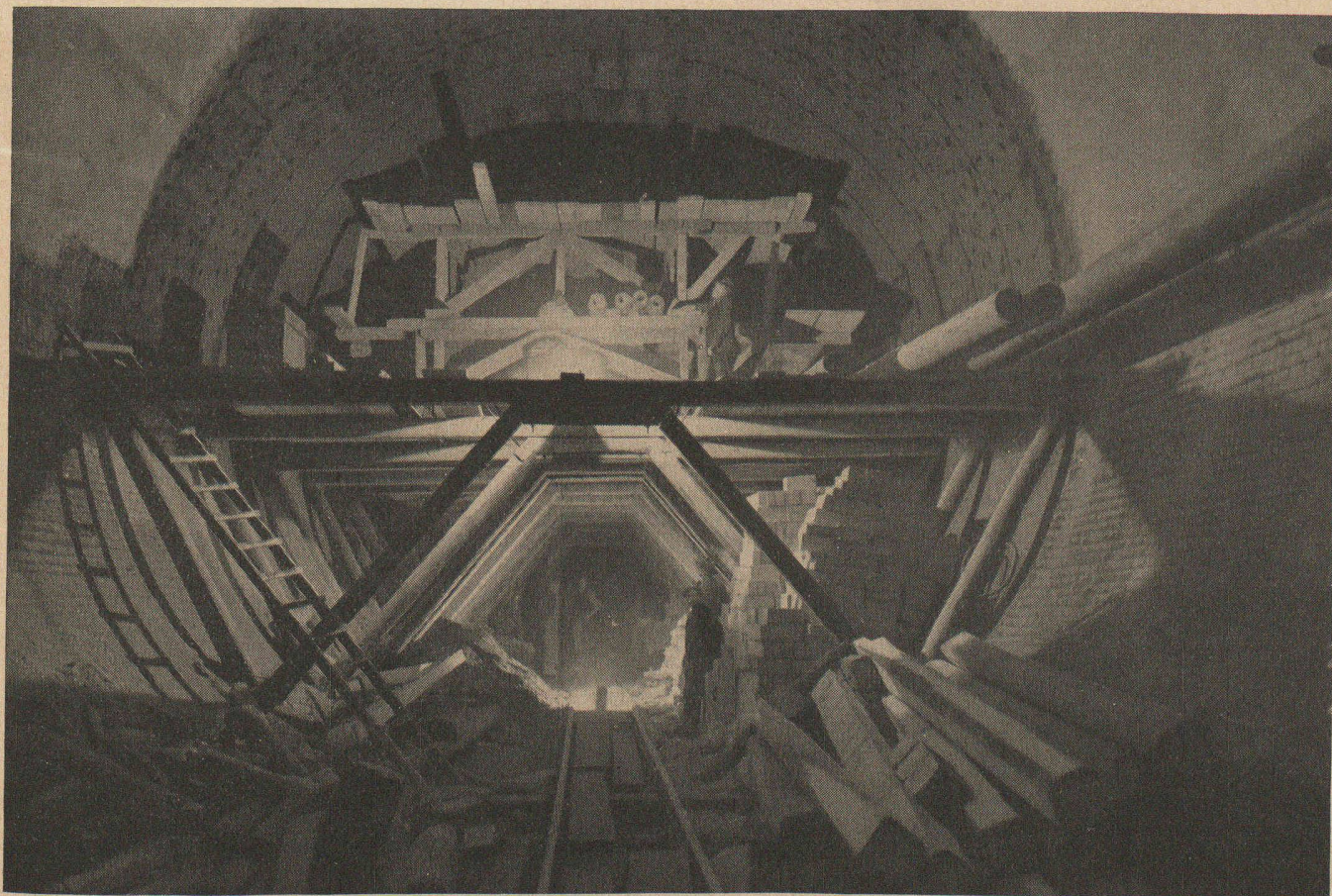
Usine électrique de Lavey. — Revêtement étanche de la galerie d'amenée sous pression, exécuté en asphalte souple « système Hirschy ».
