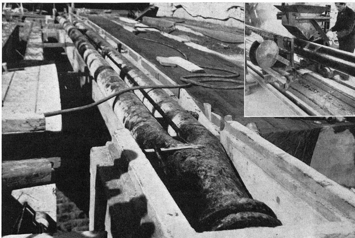
Conduite d'aduction d'eau de la Ville de Genève ; traversée du nouveau Pont de l'Ecu.
