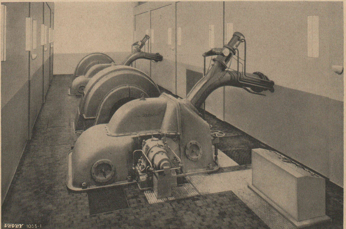
Vue de la salle des machines de la Centrale de Sassello des Forces motrices de la Calancasca S. A. Les deux turbines de 14 130 ch chacune ont été livrées, avec leurs régulateurs, par les Ateliers de Constructions Mécaniques de Vevey S. A.
