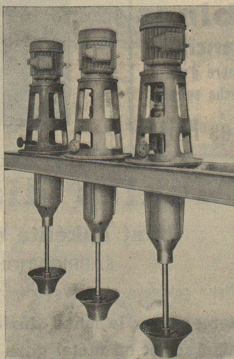
Hélices turbo-sécheur
