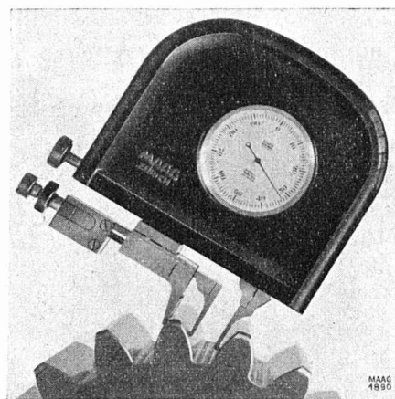
Appareil MAAG, type TME-2 à mesurer le pas normal des engrenages
