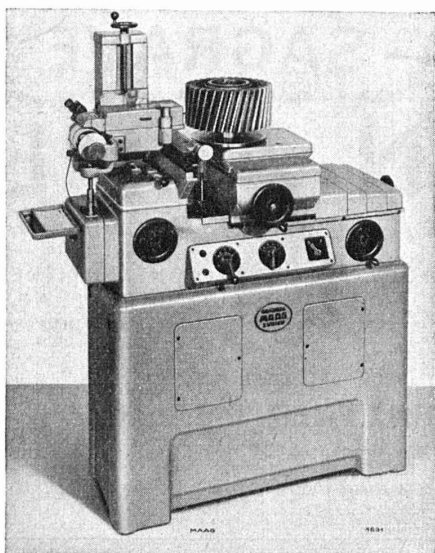
Machine MAAG à contrôler les engrenages, type PH-60
