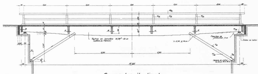
Coupe longitudinale
