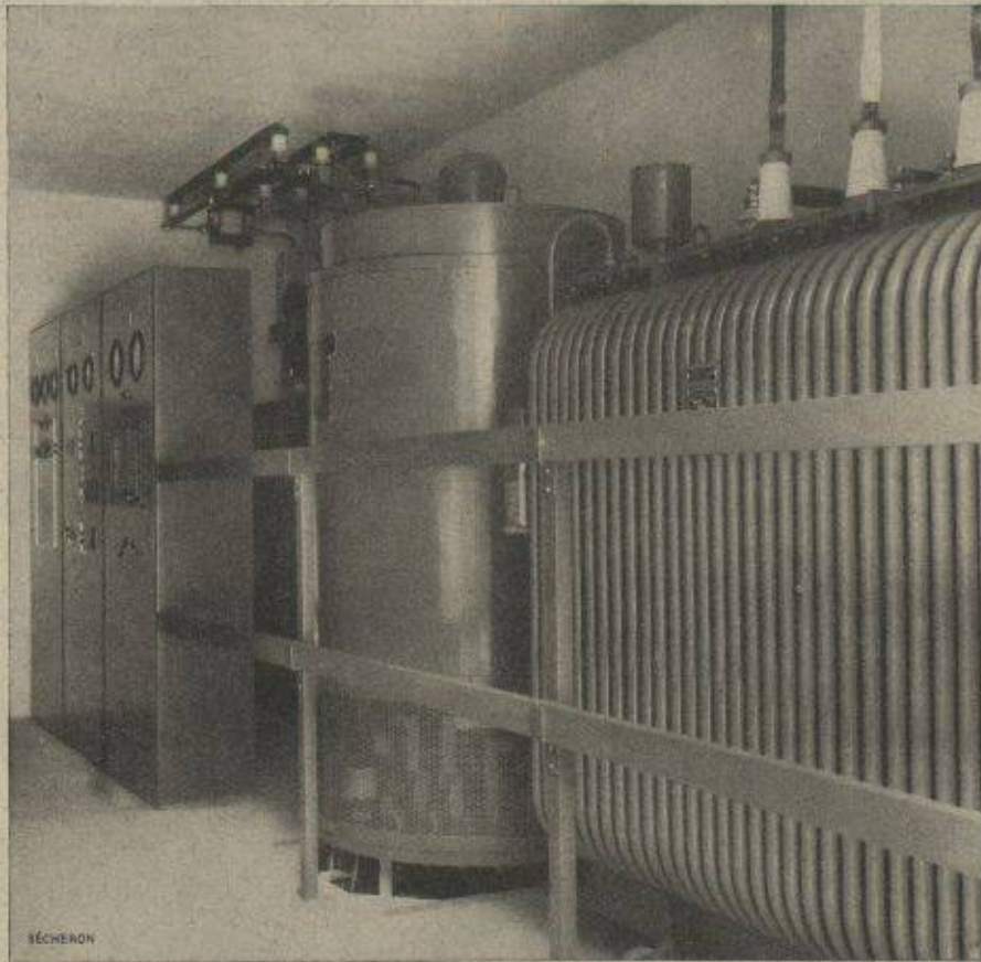
E. W. Berne. — Sous-station d'alimentation du réseau des transports publics de la Ville de Berne. — Le redresseur sans pompes à vide, à atmosphère de gaz rare, débite 1000 A sous 850 V. — Commande à distance par téléphone.
