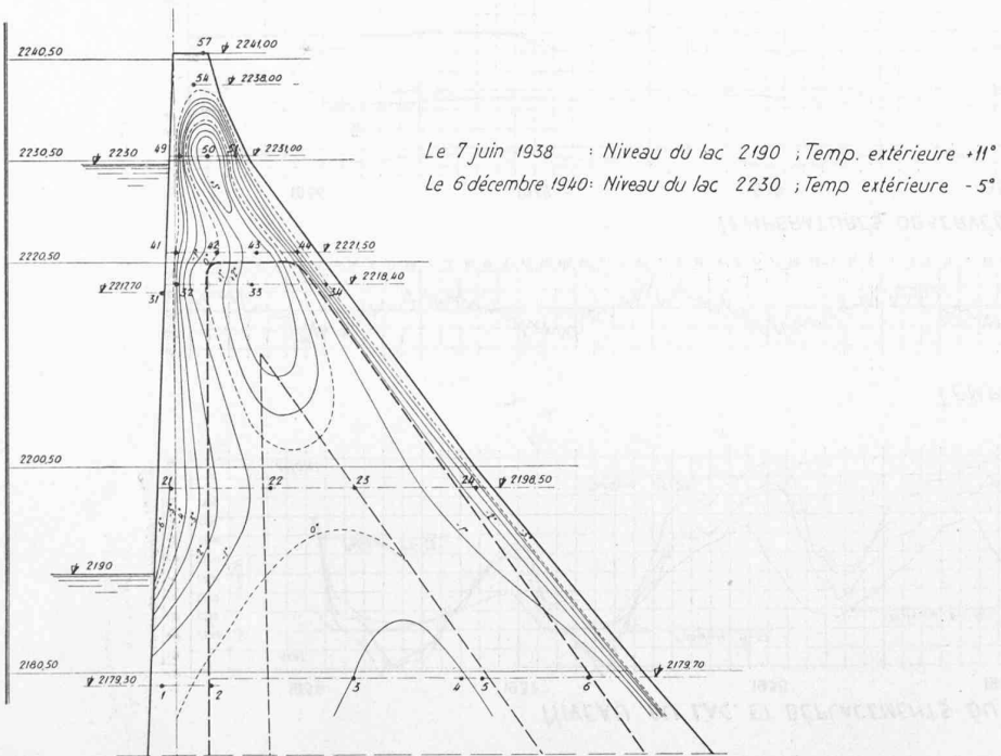
Fig. 21. — Lignes d'égal variation de température dans le plan axial du pilier 9, du 7 juin 1938 au 6 décembre 1940.
