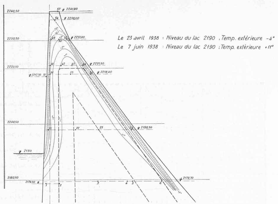
Fig. 20. — Lignes d'égal variation de température dans le plan axial du pilier 9, du 23 avril 1938 au 7 juin 1938.
