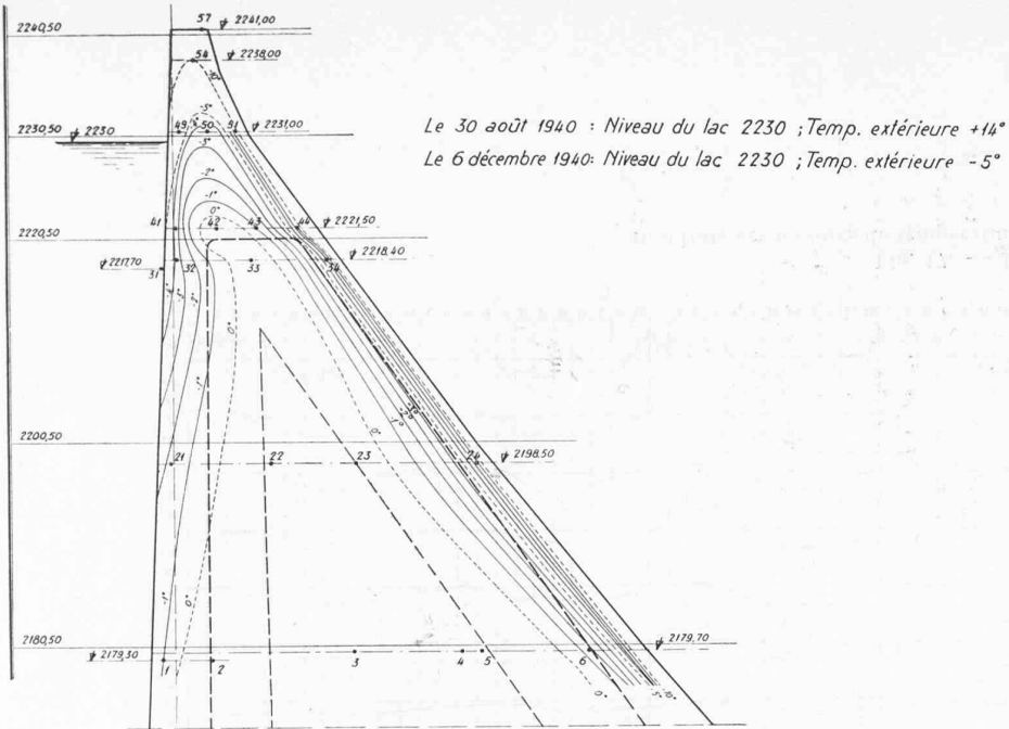
Fig. 19. — Lignes d'égal variation de température dans le plan axial du pilier 9, du 30 août 1940 au 6 décembre 1940.
