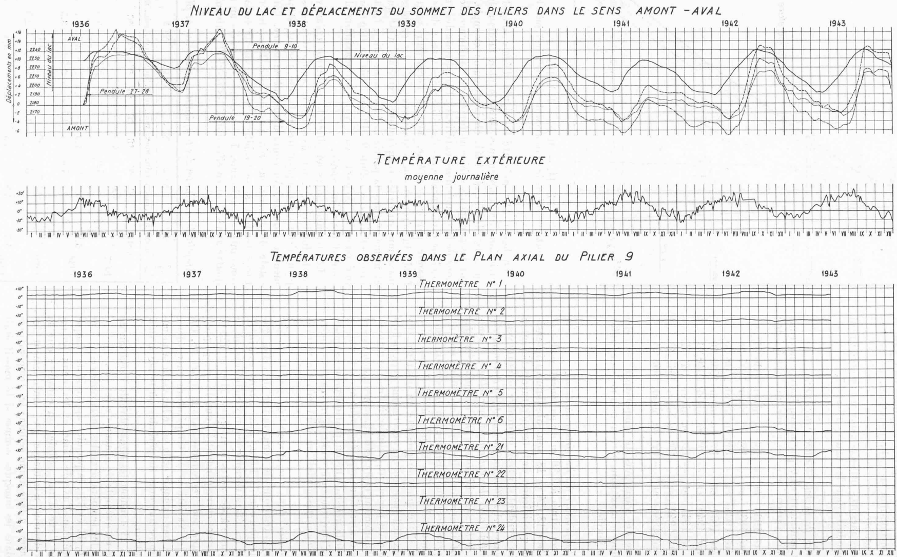
Fig. 16. — Barrage de la Dixence. Résultats des mesures de température et de déformation effectuées de 1936 à 1943.
