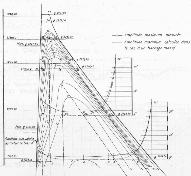
Fig. 22. — Lignes d'égal amplitude maximum des variations de température annuelles, pilier 9. — Année 1941.
