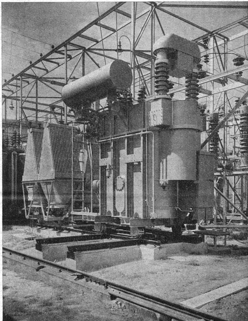
Forces motrices bernoises S.A. - Station transformatrice de Berthoud - Transformateur triphasé de 6000 KVA, 49000 \pm 1700 \pm 10 \times 504 / 16900 - 17500 V, 50 pér./s. avec insérateur de prises sous charge, manœuvrable à distance.
