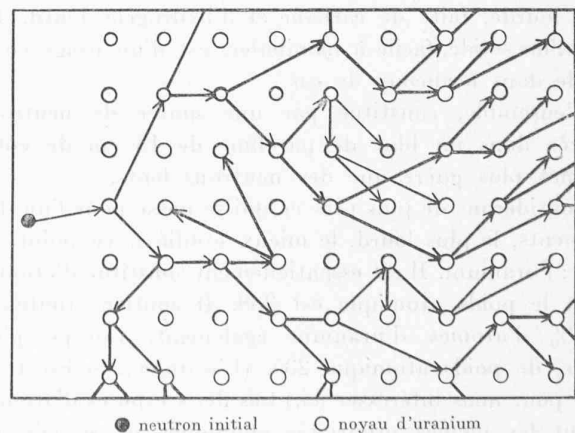
Fig. 3. — Schéma d'une réaction en chaîne. Chaque noyau qui réagit en fait réagit deux autres.
