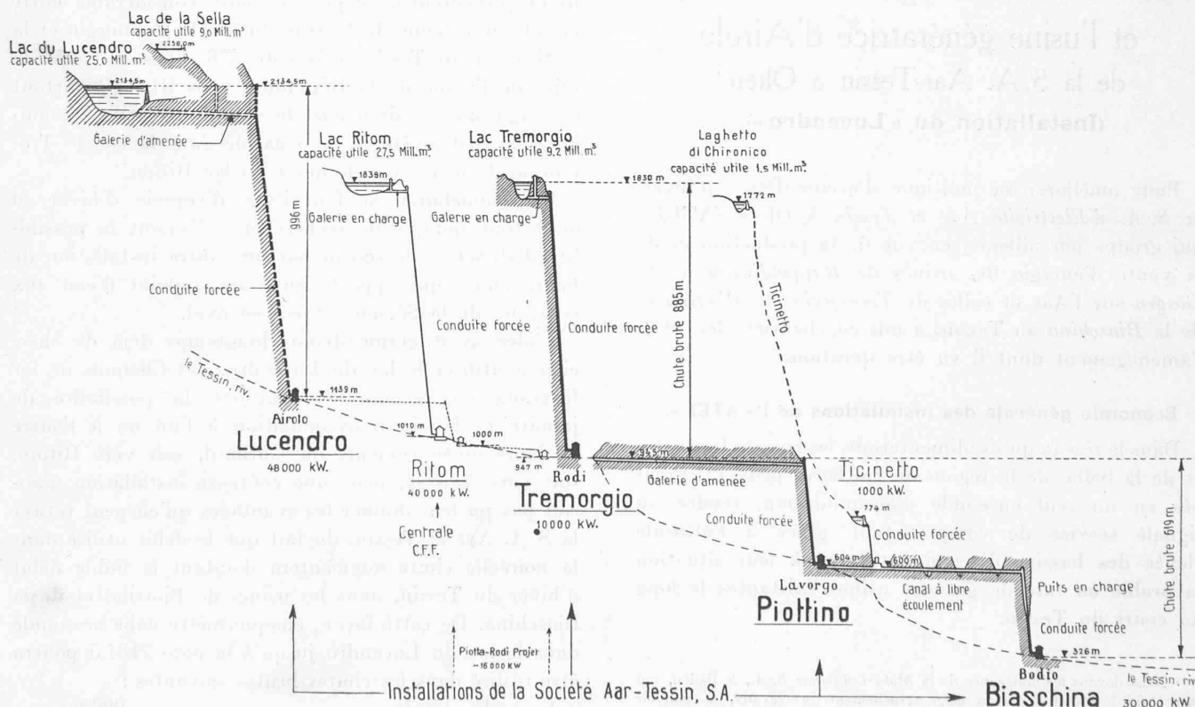
Fig. 1. — Profil en long général des installations de la Léventine.
