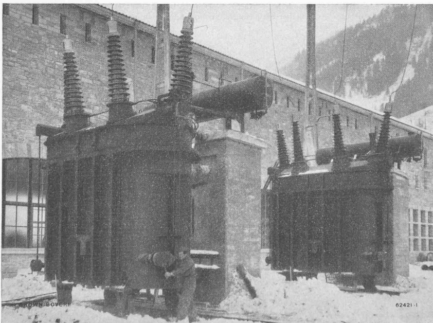
Fig. 15. — Transformateurs à haute tension triphasés à trois enroulements de 31 MVA, 11/160-145 kV.
