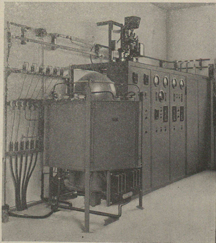
Redresseur de traction, 240 kws, 600 volts
