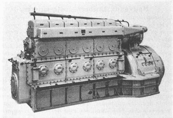
Moteur Diesel Sulzer de locomotive de 735 CV avec génératrice Oerlikon à courant continu.
