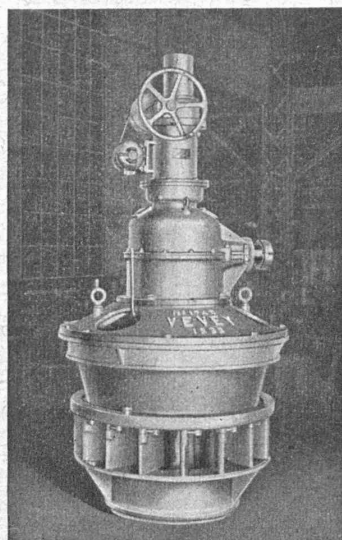
Turbine Kaplan.
