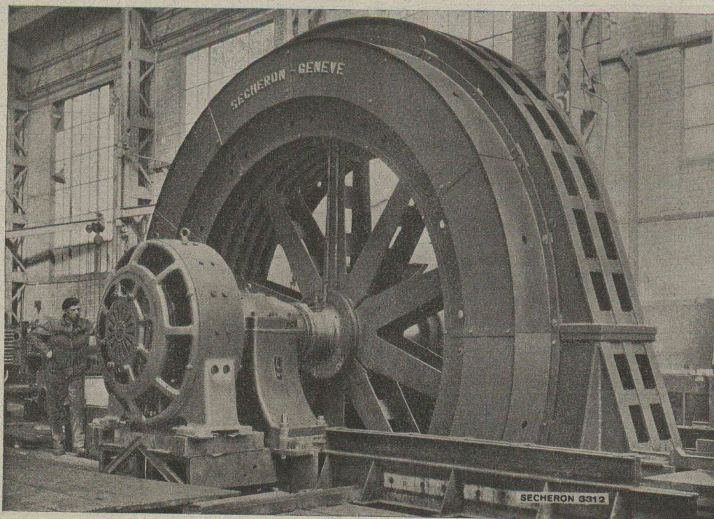
Alternateur triphasé de 7000 kVA, 150 t/min, à carcasse entièrement soudée, destiné à une grande centrale électrique de Suède. Montage pour essais en ateliers.
