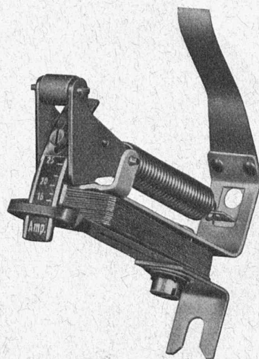
BROWN BOVERI
