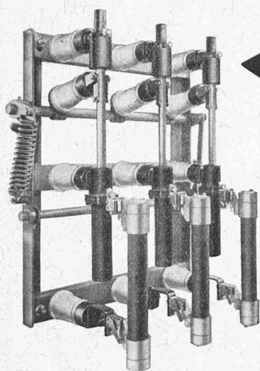
Sectionneur autopneumatique Type AS104 10 kV — 200 A.
