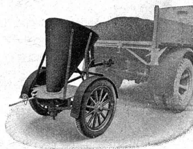
Sableuse derrière camion.
