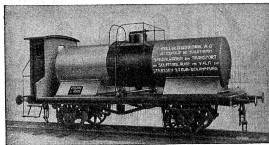
Wagon-Citerne.
