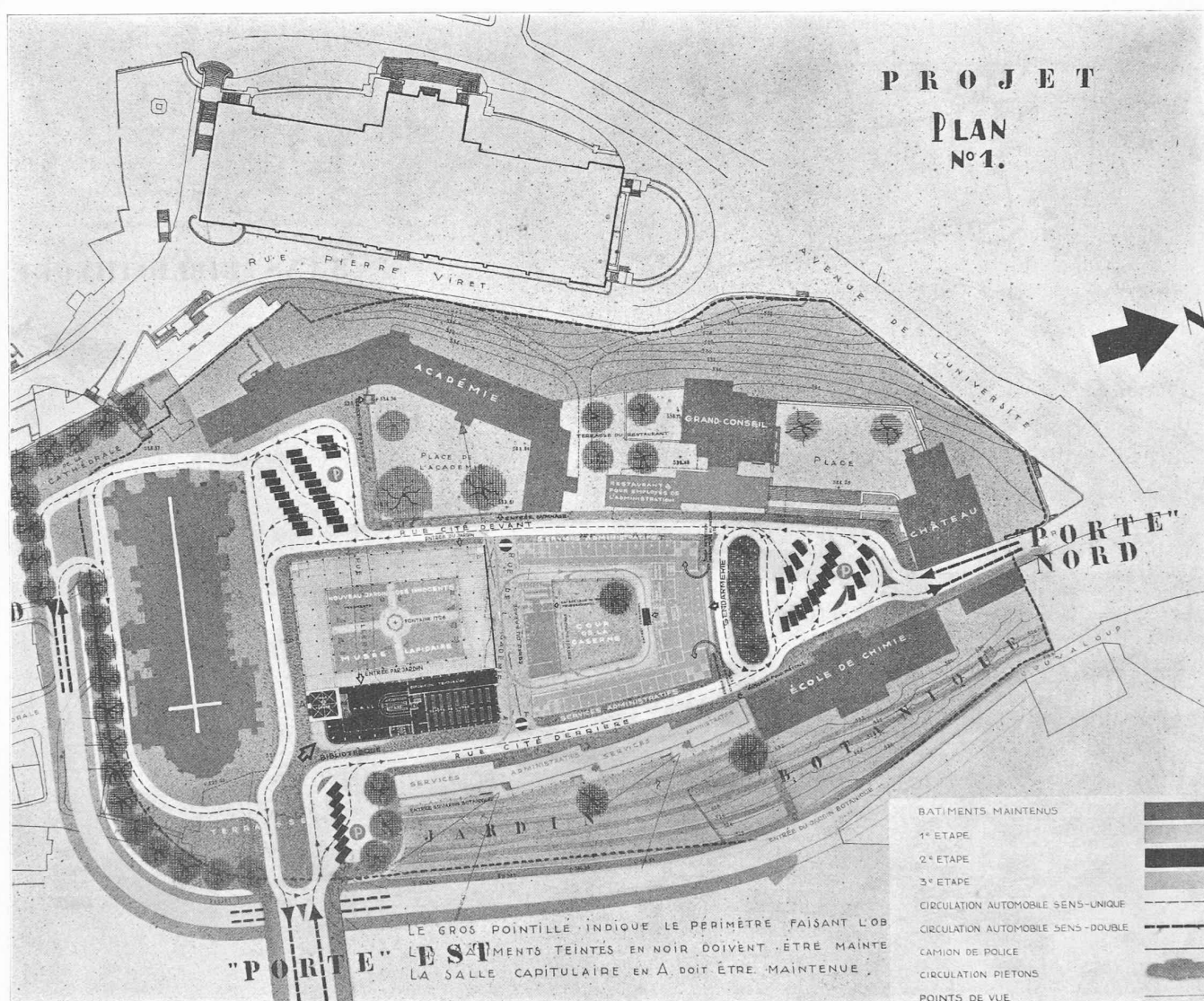
Plan général. — 1 : 2000.
