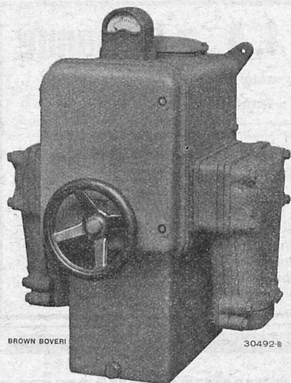
Coffret de manœuvre à déclencheurs thermiques Type MB, 250, 400 et 640 A.
