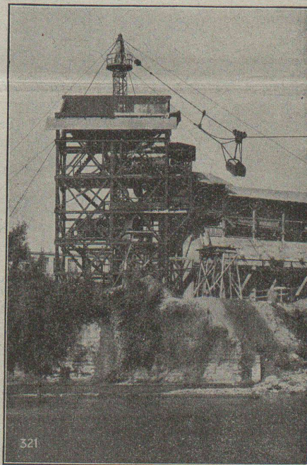
Drague à câbles sur l'Arve à Genève.
