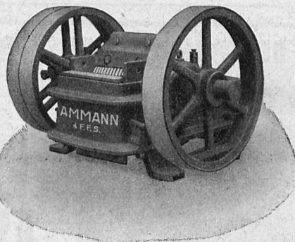
Concasseur- gravillonneur à mâchoires construit en 3 modèles pour rendements de 2 à 5 m³/heure.
