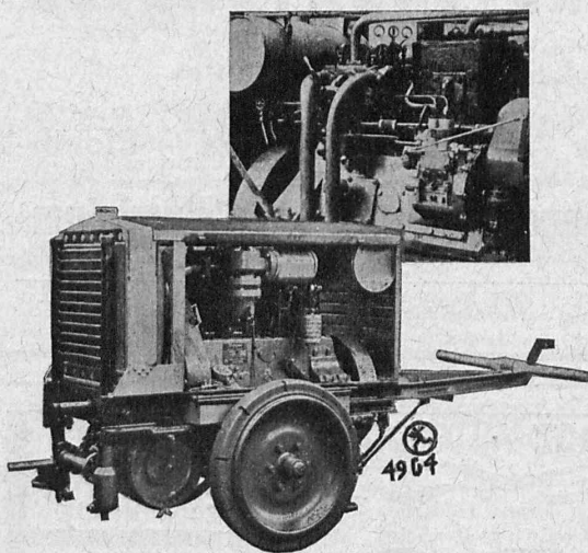
Moto-compresseur lourd type LX 26 à mazout pour l'actionnement simultané de 2 marteaux-perfora- teurs ou 2 brise-béton. Mobile, souple, économique. Installations fixes toutes puissances.
