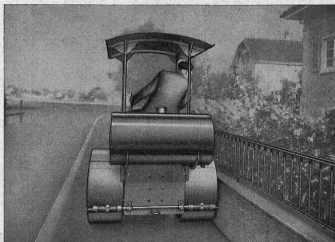
Rouleaux-moteur trijantes 3-5 tonnes, pour cylindrage de tapis, incorporation du gravillon, travaux de trottoirs. Autres modèles de 500 Kgs. à 12 tonnes.
