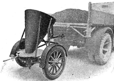
La Sableuse "Ama" pour le verglas.
