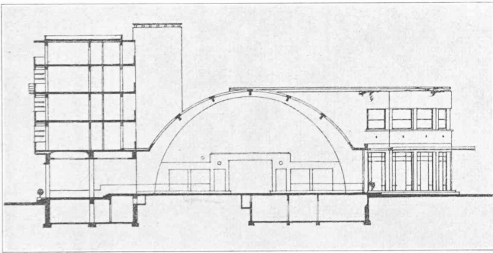
Coupe en travers. — 1 : 600.
