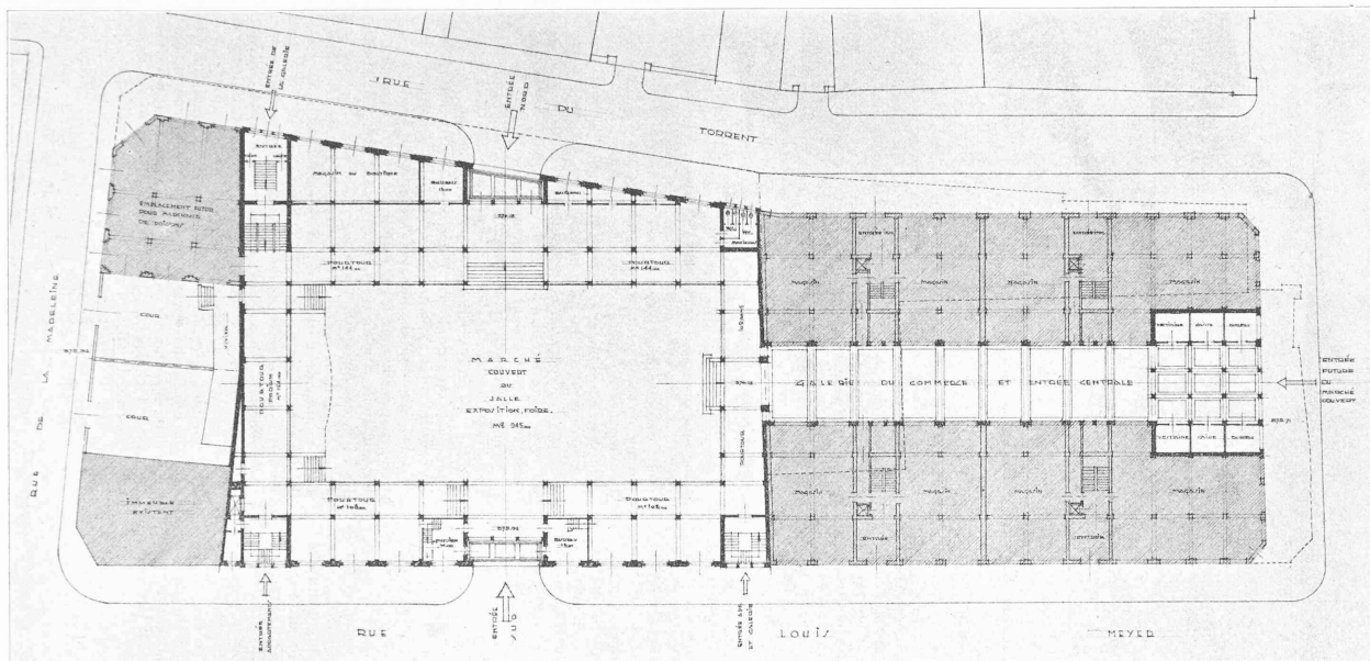
Plan du rez-de-chaussée. — 1 : 600.
