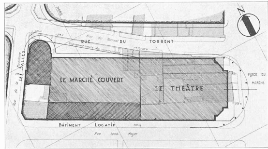
Plan de situation. — 1 : 1500.
