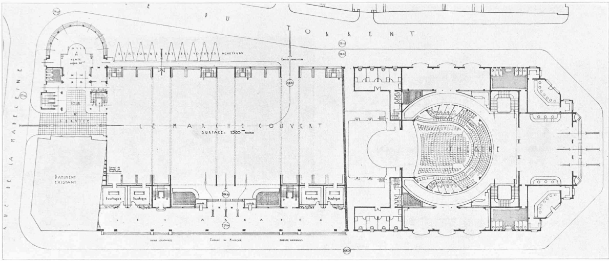
Plan du rez-de-chaussée. — 1 : 600.
