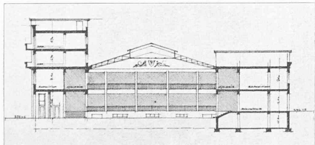
Coupe transversale 1 : 600.
