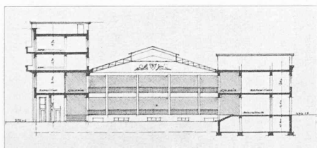
Coupe transversale 1 : 600.
