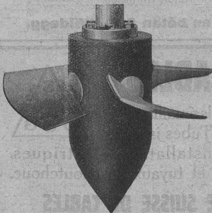
Turbine-hélice, à pales réglables.
