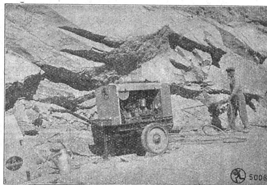
Moto-compresseur roulant LZ 20, pour 1 marteau, se distingue par sa légèreté et sa grande mobilité en même temps que sa grande robustesse.
