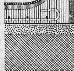
Patentierete „Isolaphon“-Unterlagsboden
