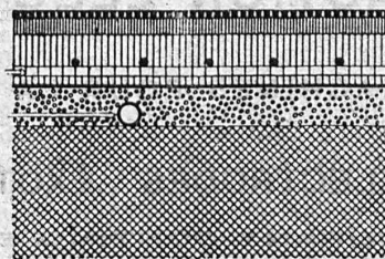
Patentierete „Isolaphon“-Unterlagsboden
