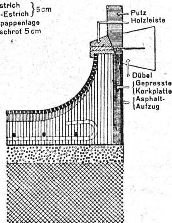
Patentierte „Isolaphon“-Unterlagsboden
