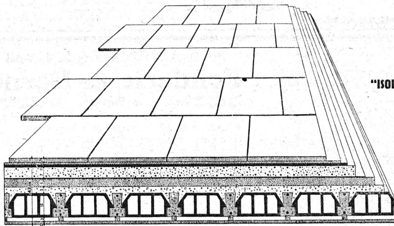
Patentierete „isoliaphon“- Flachdachkonstruktion
