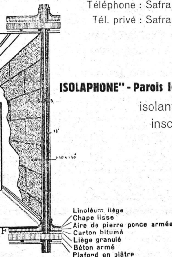
Patentierte „Isolaphon“-Leichtwände
