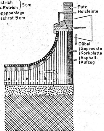
Patentierete „isoliaphon“- Unterlagsboden
