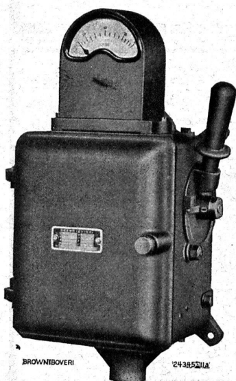
Coffret de manœuvre à déclencheurs thermiques type LC 2e pour 64 A.
