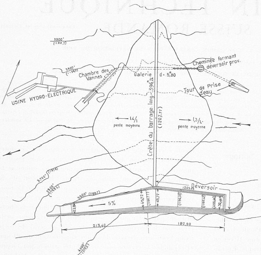
Fig. 1. — Vue en plan du barrage, avec ouvrages-annexes : déversoir, dérivation, prise d'eau, etc.
