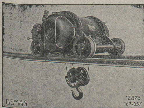
Chariot sur deux rails.
