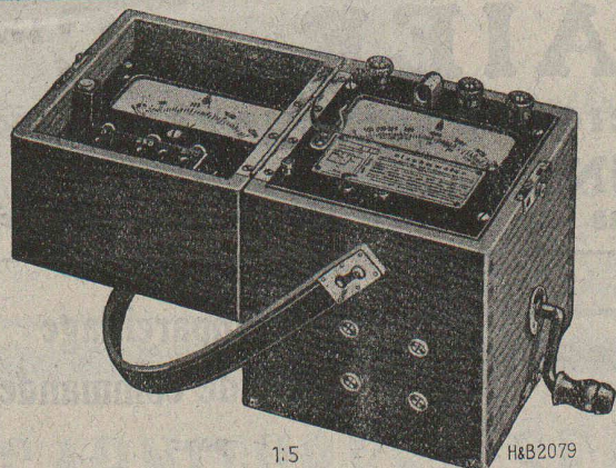
1:5 H&B2079 Mesureur d'isolement avec voltmètre.
