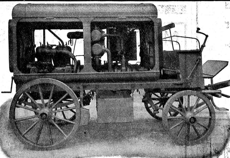
Moto-Compresseur sur char.
