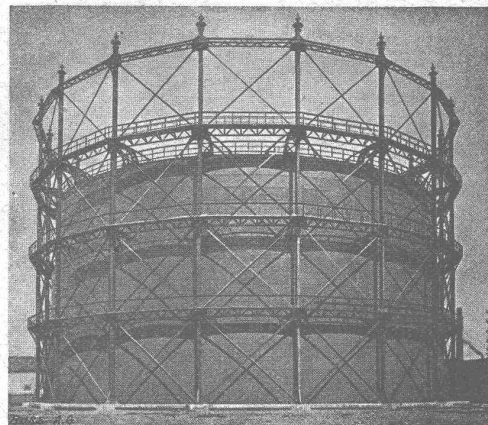
Gazomètre d'une contenance de 50,000 m³.
