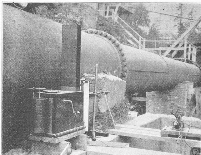
Fig. 3. — Vue arrière de l'appareil Gibson.
