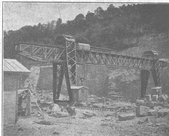
Pont roulant électrique pour carrières. — Force : 80 tonnes.
