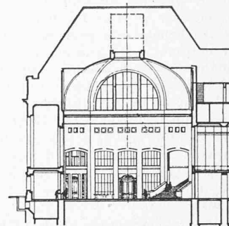
Coupe en long du hall. — 1 : 800.
