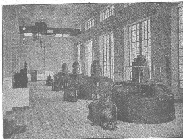
Usine de la Jagne. (Entreprises Electr. Fribourgeoises) 4 turbines de 7800 ch. chacune. Châte : 105-120 m. Vitesse : 500 t/m 1
