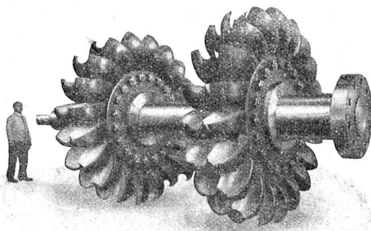
Roues motrices turbines Pelton 14300 HP. de l'usine d'Amsteg (C. F. F.)
