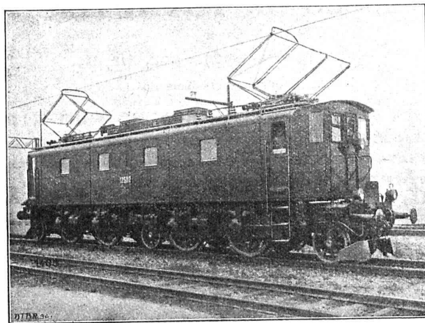
LOCOMOTIVE « SÉCHERON » TYPE 1B1 + 1B1 2'400 HP. pour la ligne du Saint-Gothard des Chemins de Fer Fédéraux Suisses.
