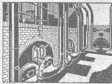
Installation de soufflerie sous grille « Foehn » pour combustibles pauvres
