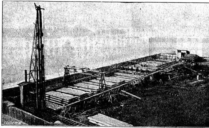
Hôtel des Postes, Saint-Gall. Sonnette à vapeur et dépôt de pieux en béton armé, système Zublin.
