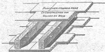
Plafond-hourdis armé s/lolives en bois.
