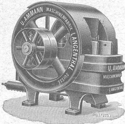
Concasseur fixe.
